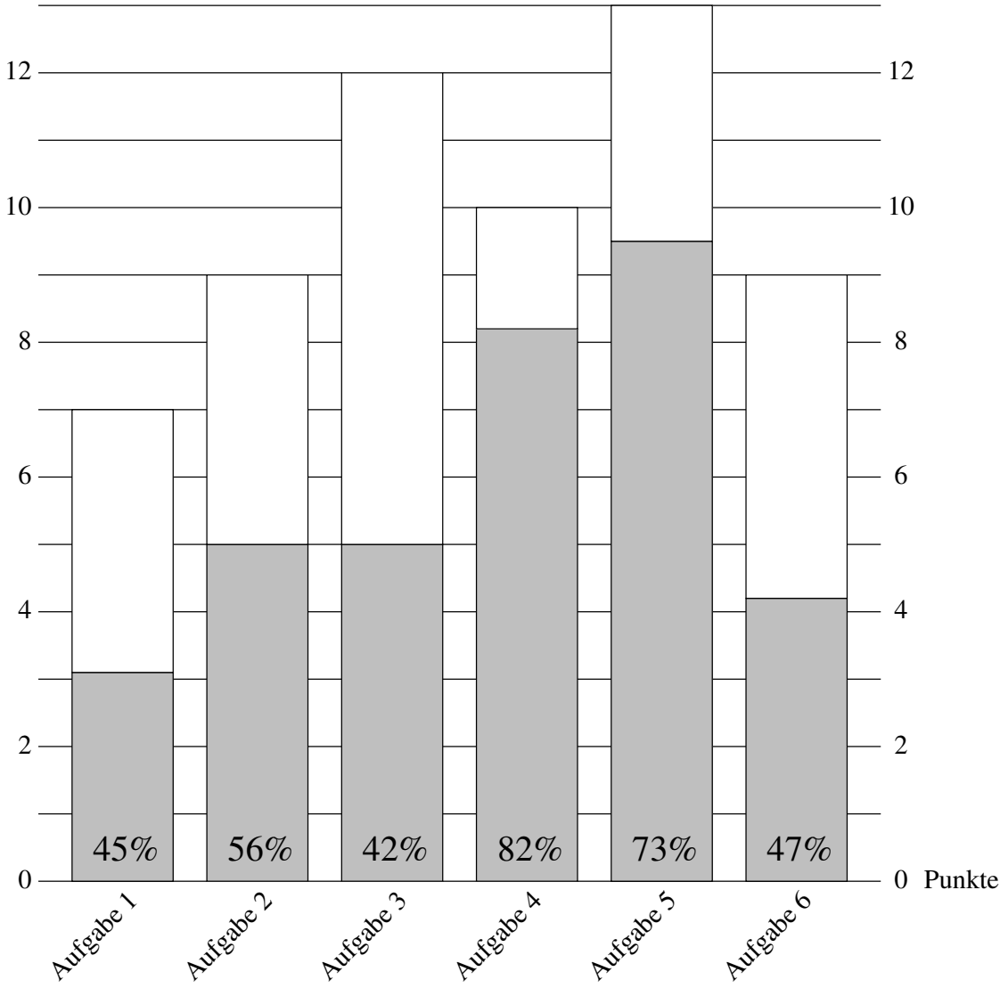
durchschnittlich erreichte Punkte pro Aufgabe:
